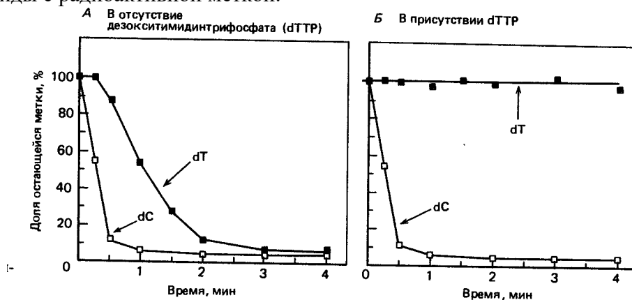
Рис. 2. Коррекция ДНК-полимеразой I в отсутствие (А) и в присутствии (Б) дТTP.
